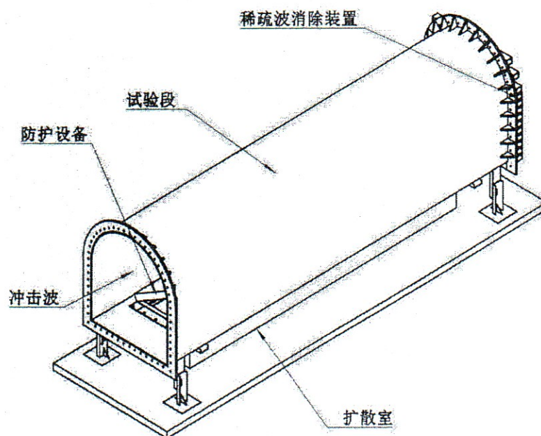
图 B. 3 水平安装防护设备固定方式示意图
