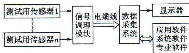
图C.2 抗性性能测试系统工作原理示意图
