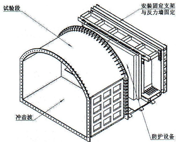
图 B. 2 大型型防护设备固定方式示意图
