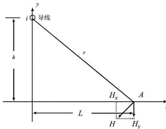
图 8-3 磁场向量图
