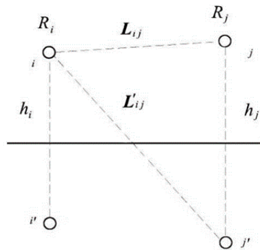
图 8-1 电位系数计算图
